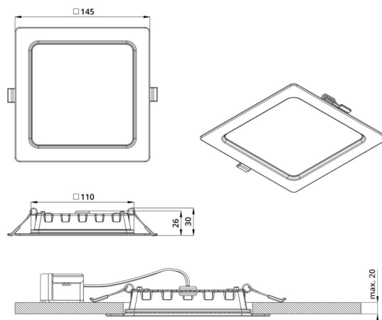
Габаритный чертеж
